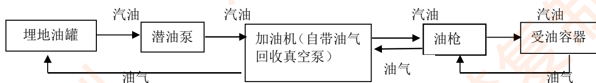
图 2.7-5 乙醇汽油加油工艺流程简图
